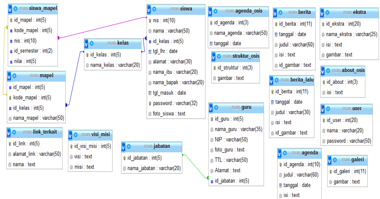
Gambar 3.5 Rancangan Database
