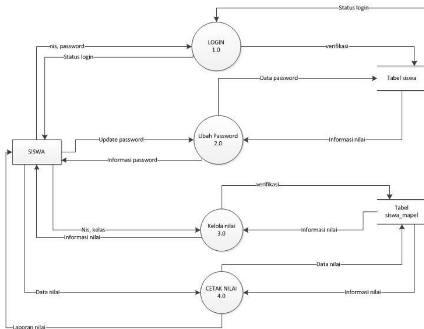
Gambar 3.2 DFD level 1 siswa
