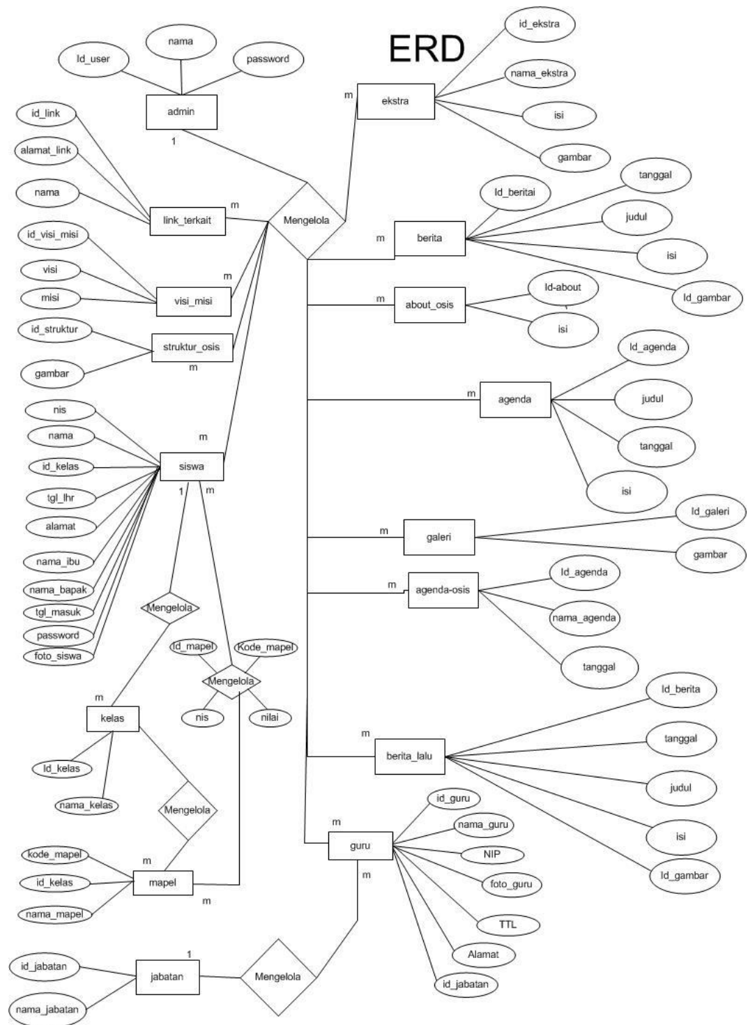
Gambar 3.3 ERD
